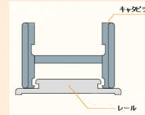
レール断面
