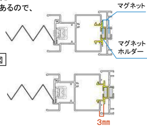
戸先部分の断面図
